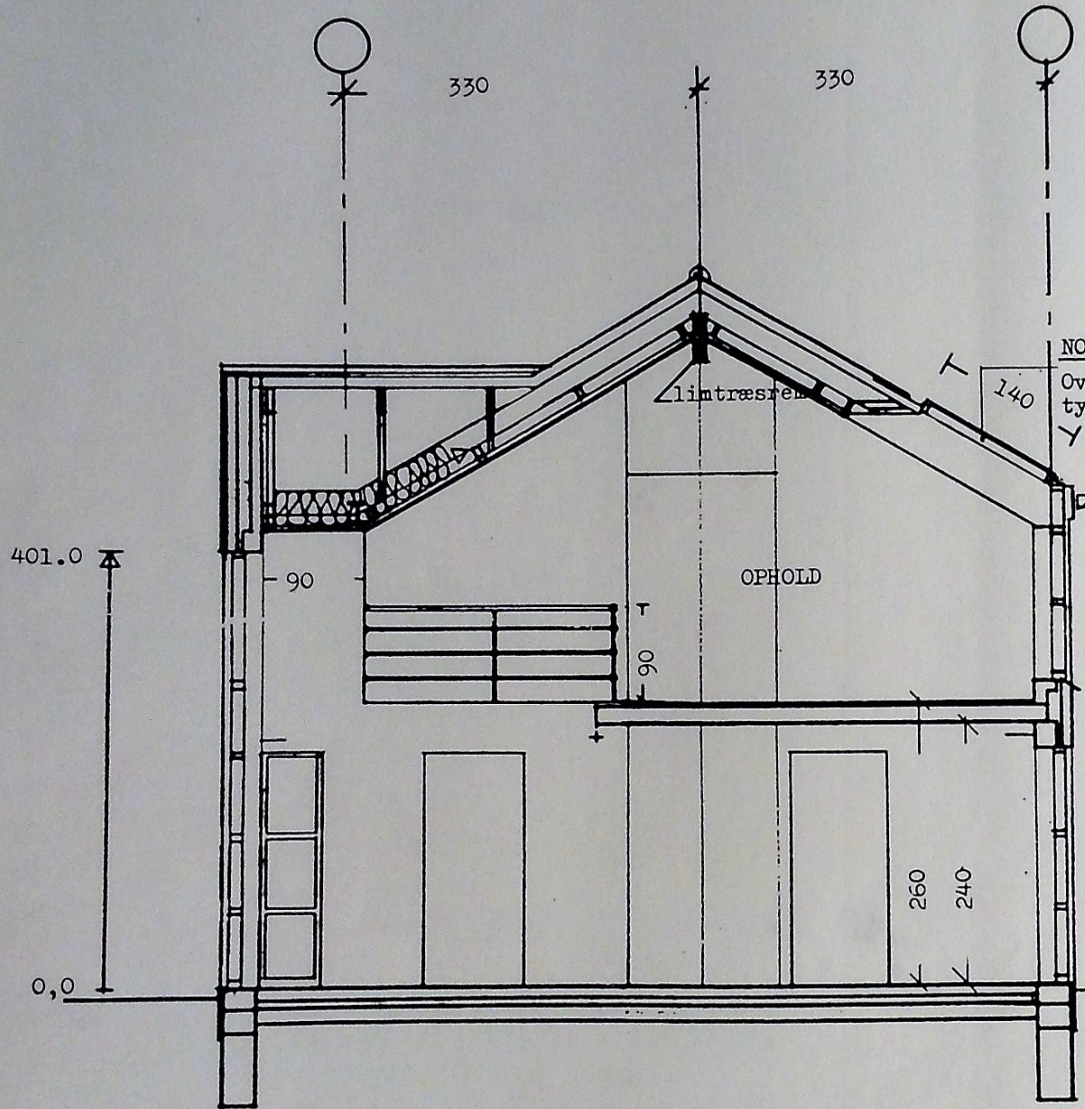
Snit G-G
