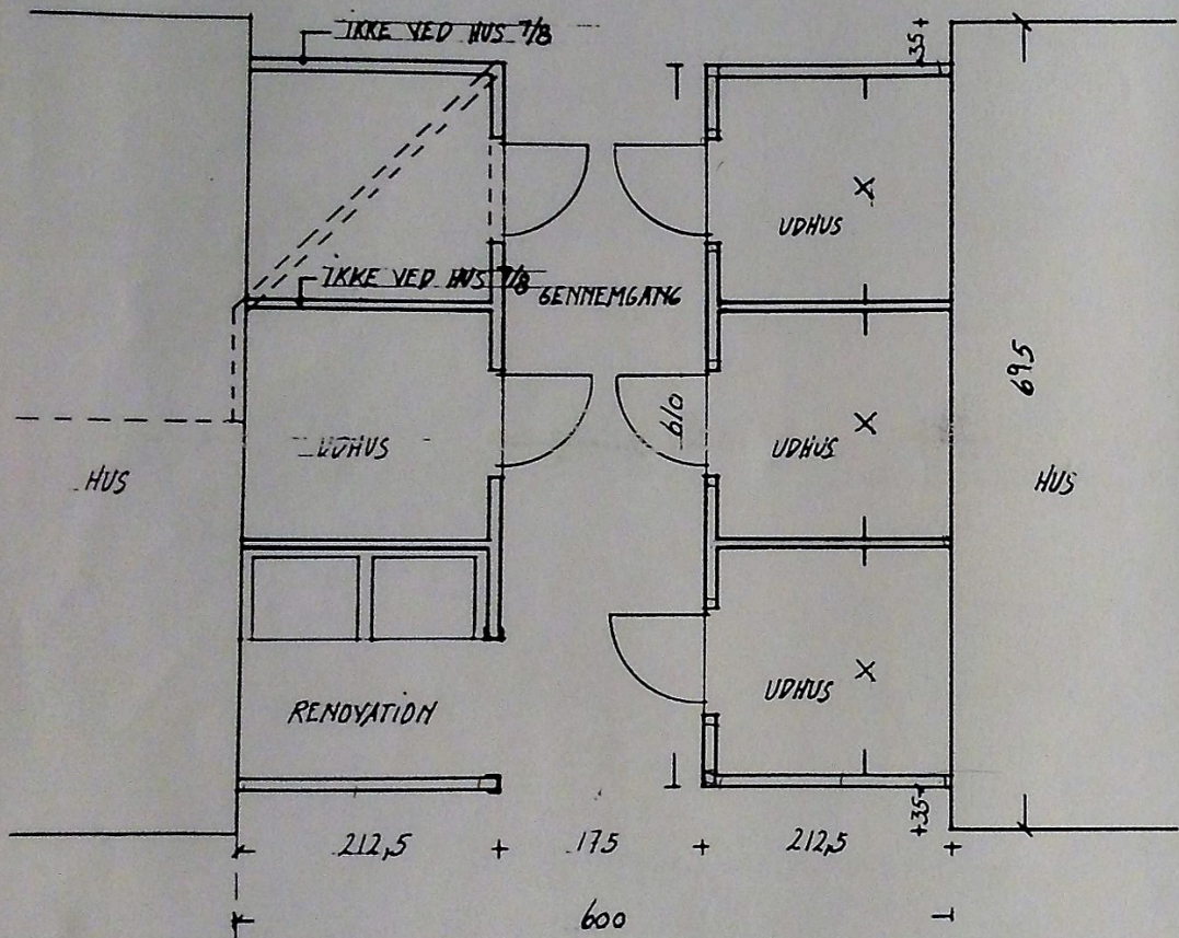
DOBBELT UDHUSSEKTION
