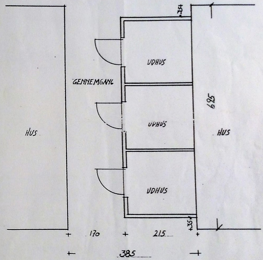
ENKELT UDHUSSEKTION
